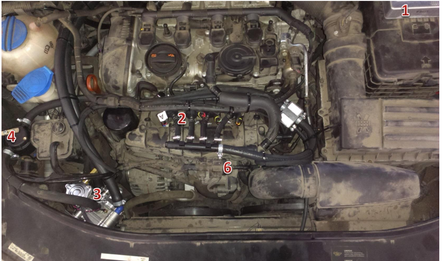
1-sterownik/ECU Zenit Direct, 2-wtryskiwacze gazu/gas injectors, 3-reduktor/reducer, 4-filtr fazy lotnej/gas phase filter, 6- króciec podciśnienia/vaccum nozzle
