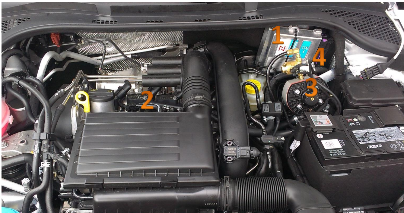
1-sterownik/ECU Zenit Direct, 2-wtryskiwacze gazu/gas injectors, 3-reduktor/reducer, elektrozawór z filtrem fazy ciekłej/electrovalve with liquid gas phase filter, 4-filtr fazy lotnej/gas phase filter
