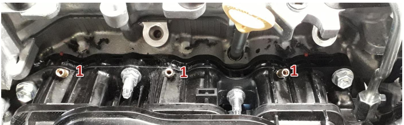
1-dysze wtryskiwaczy gazu/gas injector nozzles
